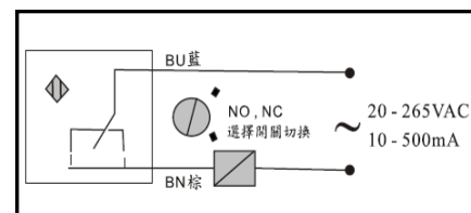
AC 二線式
